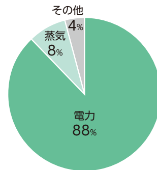
CO 2 排出量種類別割合 2018年度
