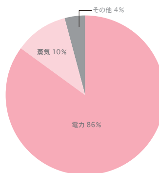
CO 2 排出量種類別割合 (2015年度)
