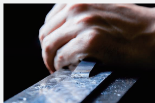
きさげ加工
